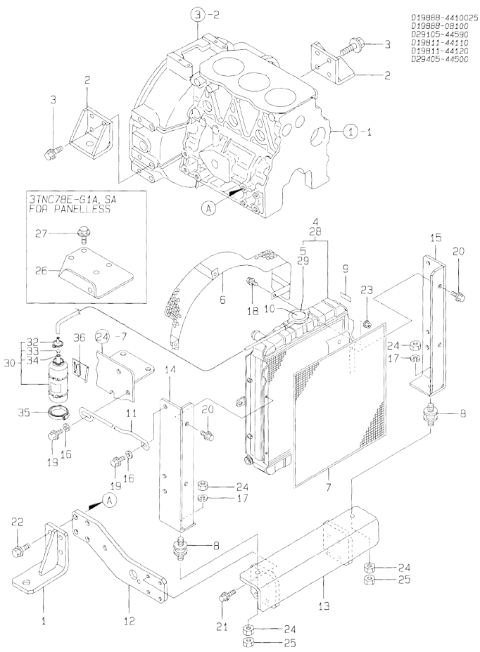
Fig.11. RADIATOR
